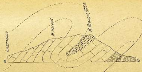
Fig. 67. — Sezione attraverso il M. Narunt.
