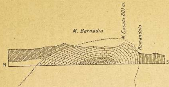
Fig. 14. — Sezione attraverso il M. Bernadia.
