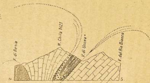
Fig. 92. — Sezione attraverso la Val di Uceca.
