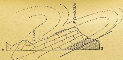
Fig. 66. — Sezione attraverso il M. Covria.
