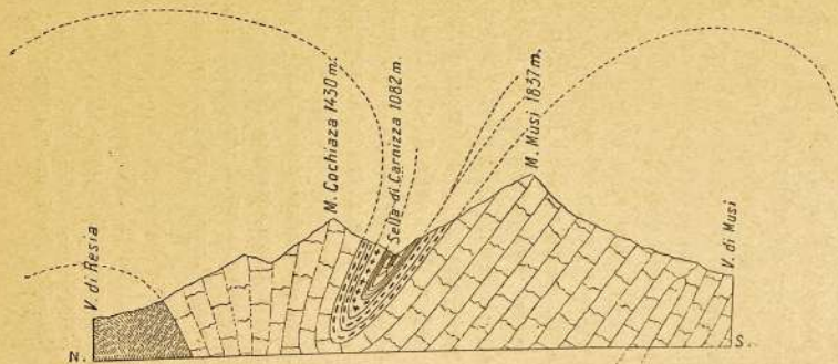
Fig. 91. — Sezione attraverso la sella di Carnizza.
