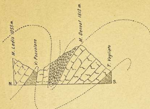
Fig. 68. — Sezione attraverso la Val Pozzolons.
