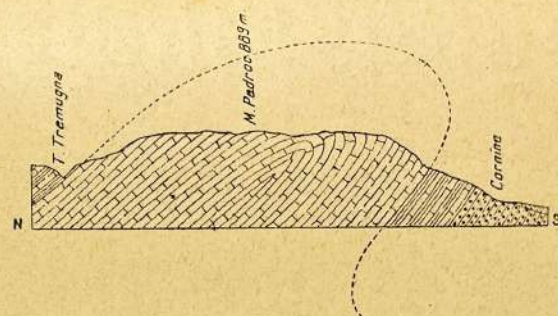
Fig. 13. — Sezione attraverso il M. Pedroc.
