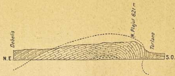
Fig. 15. — Sezione attraverso il M. Plajul.
