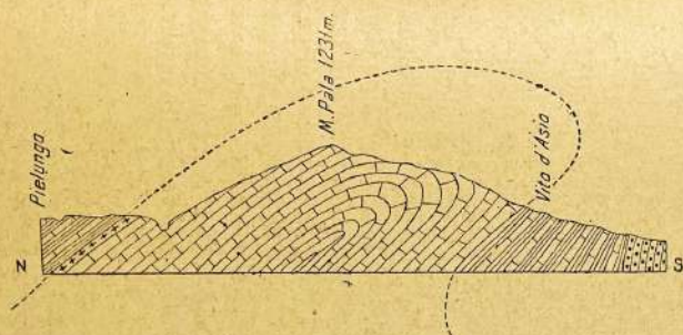
Fig. 12. — Sezione attraverso il M. Pala.
