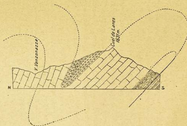
Fig. 69. — Sezione attraverso il Cuel de Lanes.
