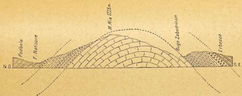
Fig. 16. — Sezione attraverso il M. Mia.
