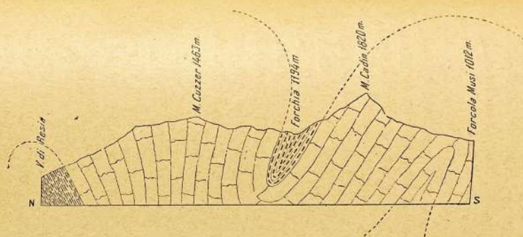
Fig. 90. — Sezione attraverso i monti Cadin e Cuzzer.
