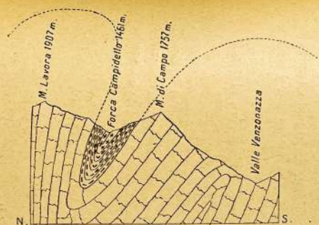
Fig. 89. — Sezione attraverso la Forca Campitello.
