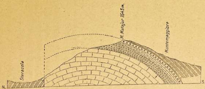
Fig. 17. — Sezione attraverso il M. Matajur.
